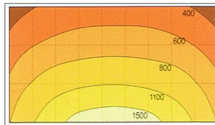
DF830D12を使用。 W900xD300xH300の水平面照度(Lx)
